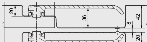
Exemple d'utilisation 656S42/656S20
