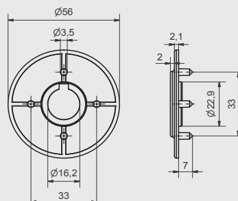
Rosace de recouvrement R3495
